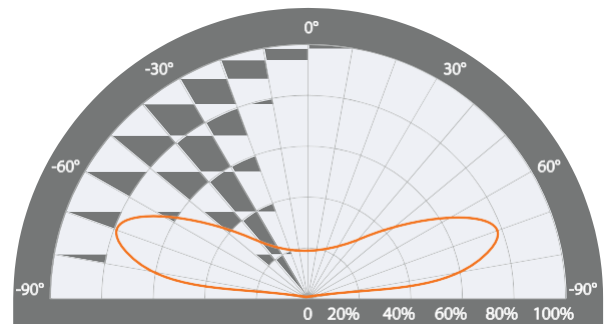
Latitudinal (vertical angle) Polar Radiaton Pattern
